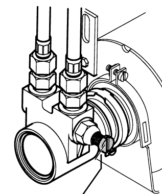
Z = Pumpendruck-Regulierungsschraube
